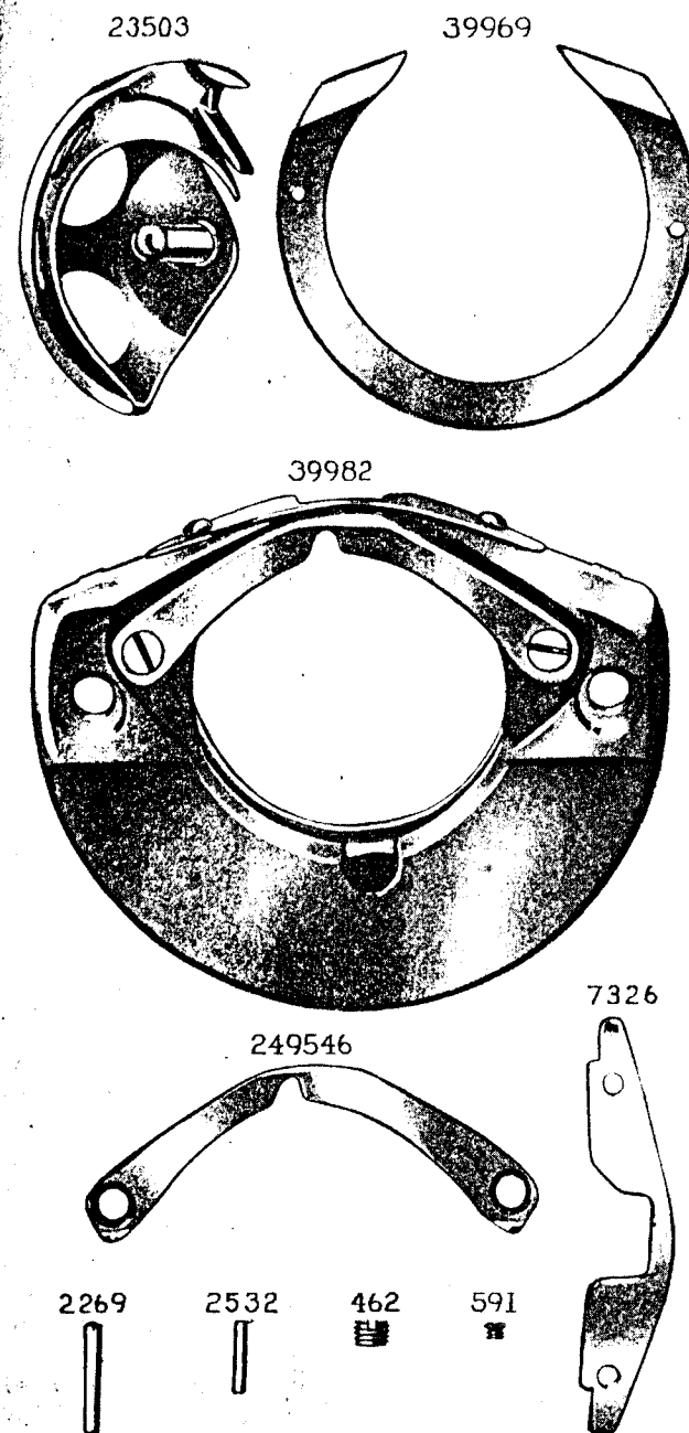
PLATE 14978—FULL SIZE
